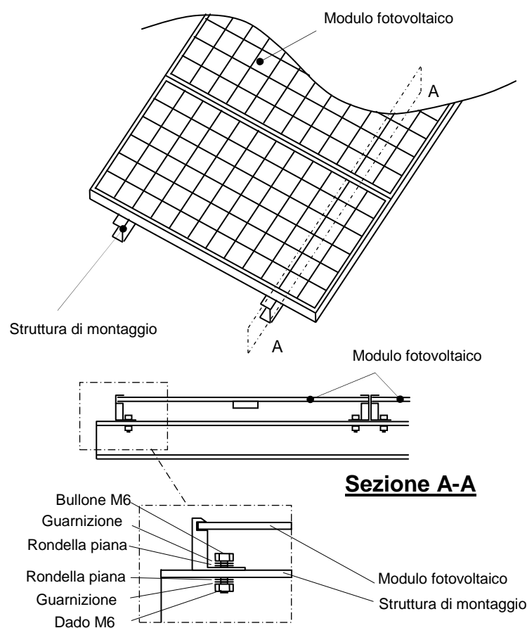
Figura 1: Installazione
