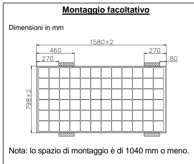
Figura 2-3: Montaggio facoltativo
