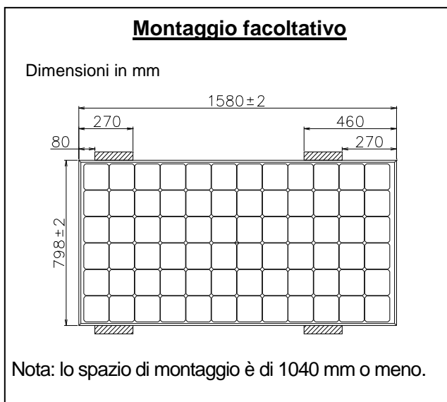
Figura 2-2: Montaggio facoltativo
