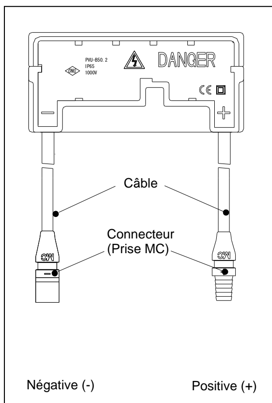
Figure 3: Configuration de la boîte de connexion
