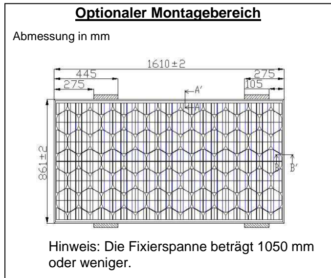
Abb. 2-3: Optionaler Montagebereich
