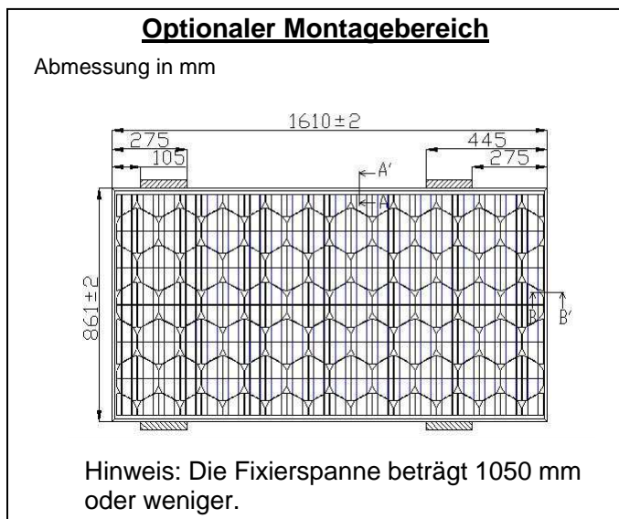
Abb. 2-2: Optionaler Montagebereich
