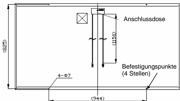
Abb. 2-1: Abmessungen
